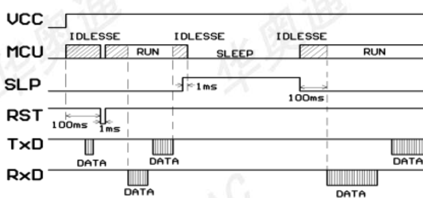
休眠功能时序图
